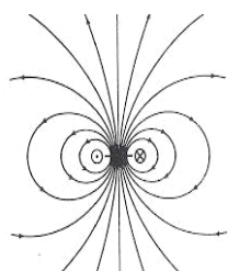
Electromagnétisme
