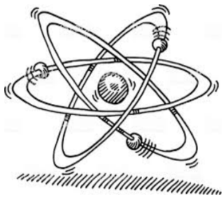
Energie cinétique
