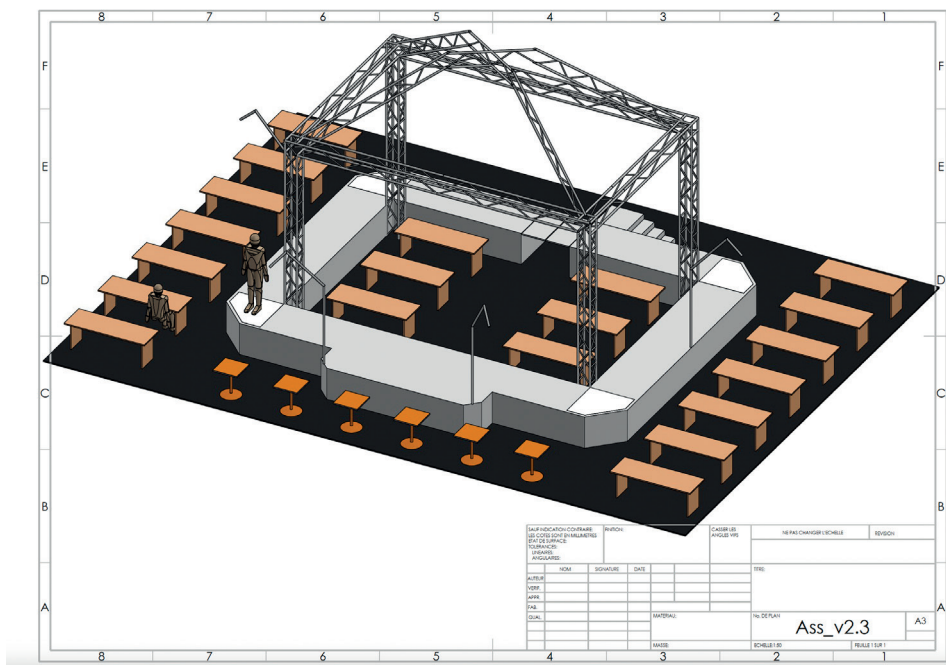
Axonométrie 1/50 e
